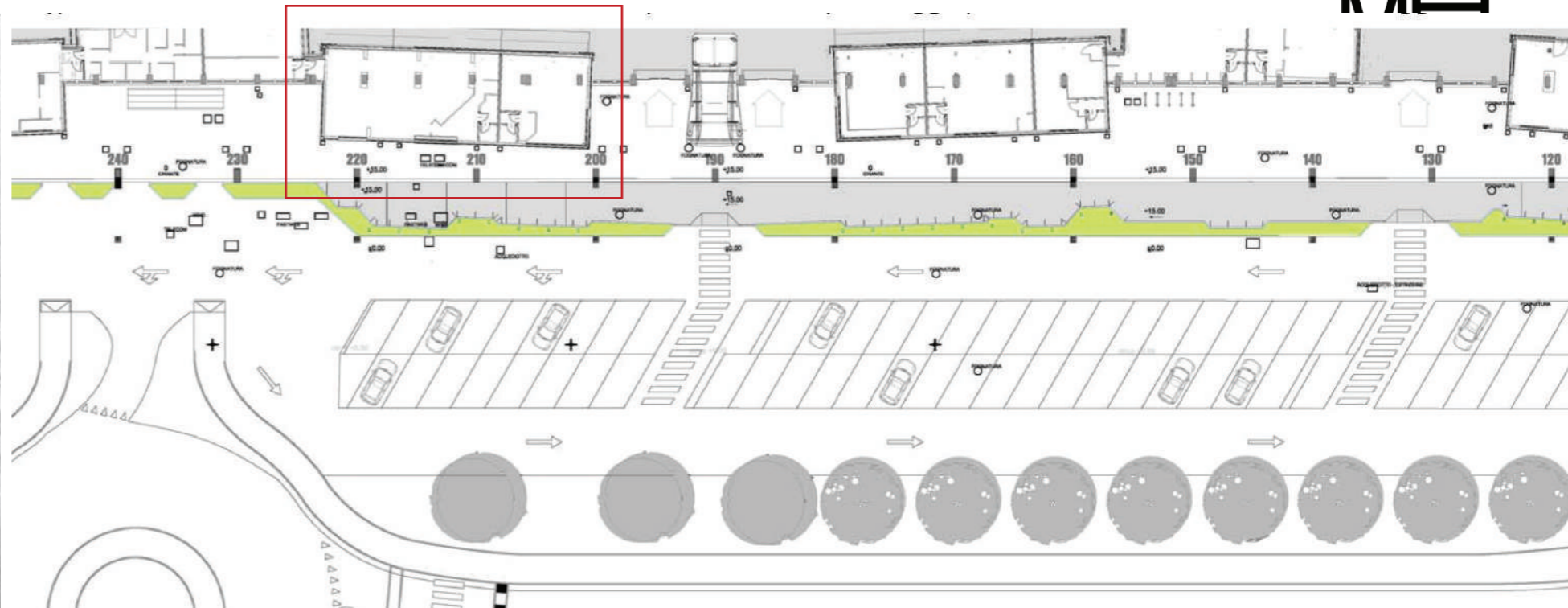
Planimetria generale ed individuazione area di intervento
